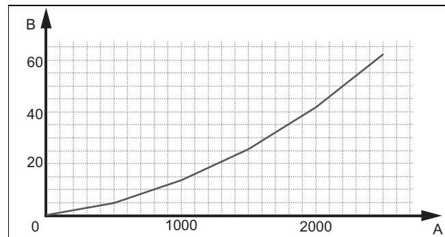
A Caudal en el circuito de agua caliente sanitaria (l/h) B Pérdida de presión (kPa)
