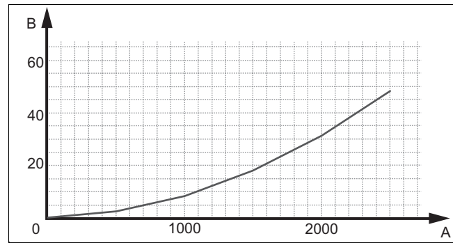
A Caudal en el circuito del edificio (l/h) B Pérdida de presión (kPa)
