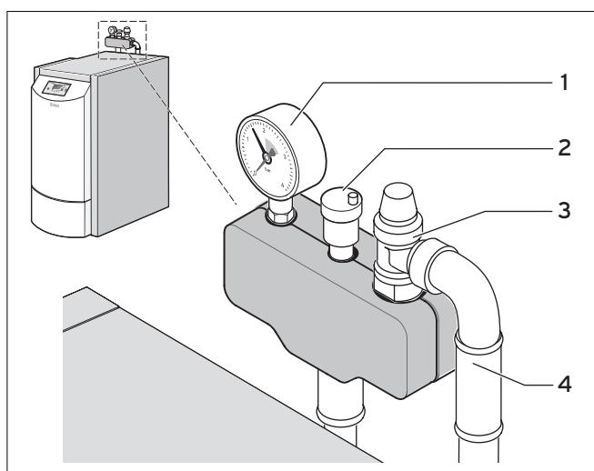
Fig. 4.10 Consulta de la presión de llenado (aquí: Grupo de seguridad Vaillant)
