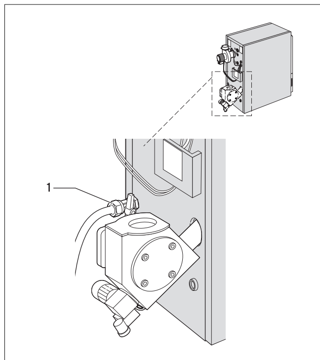
Fig. 4.11 Llenar la instalación de calefacción
