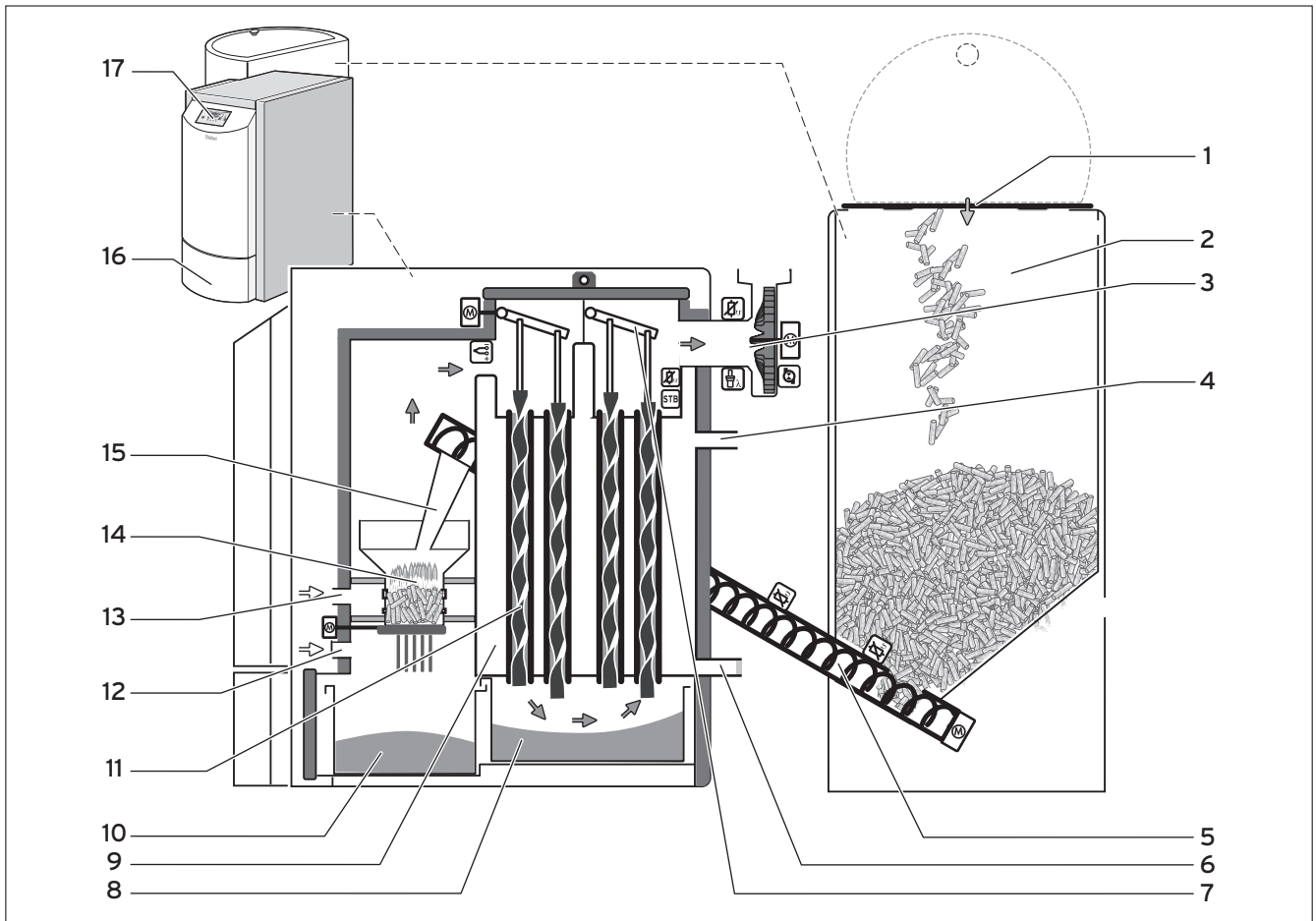
Fig. 3.1 Principio de funcionamiento de la caldera de pellets
