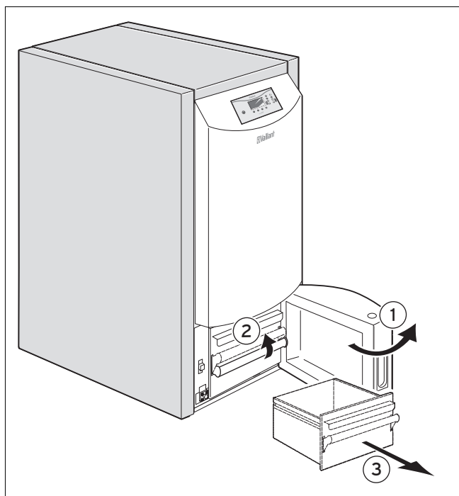
Fig. 4.7 Extracción del depósito de cenizas de dos partes
