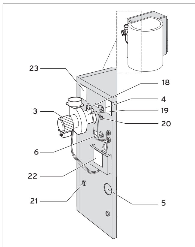
Fig. 3.2 Vista posterior de la caldera de pellets con descarga mediante tornillo sinfín
