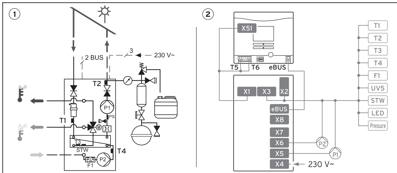
1 Esquema hidráulico
