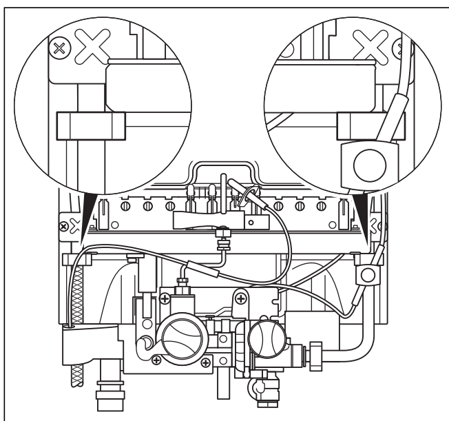
Fig. 7.4 Conexiones de agua de los serpentines del aparato
