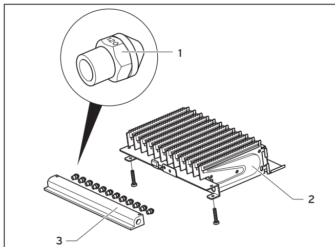
Fig. 6.3 Identificación de las toberas
