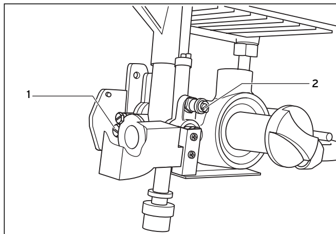
Fig. 6.4 Tobera de medición para la presión del quemador
