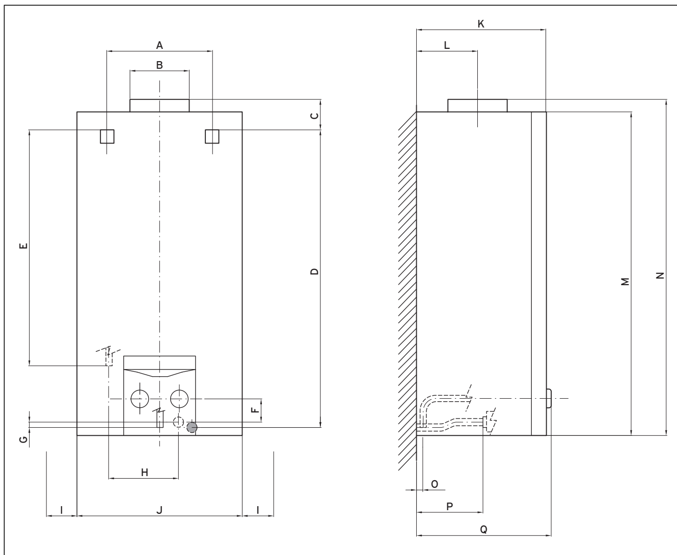
Fig. 4.2 Dimensiones mini 14-O/O XF gas butano, gas natural
