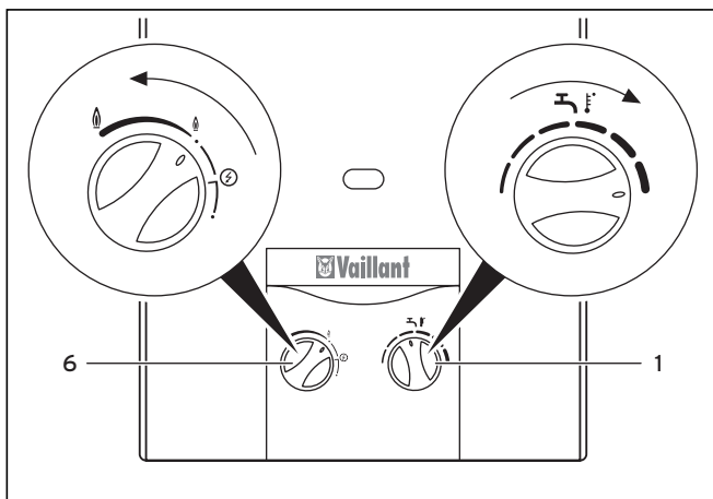
Fig. 7.5 Ajuste de temperatura y potencia máximas
