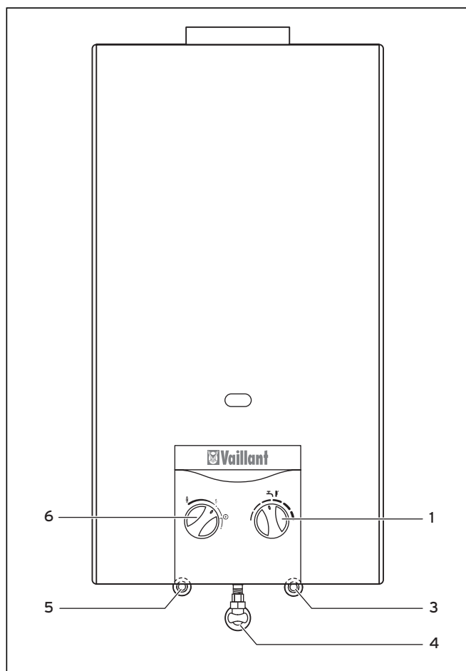
Fig. 4.1 Elementos de mando del aparato atmoMAG
