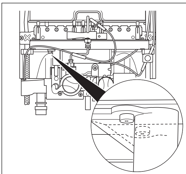
Fig. 7.2 Fijación del quemador en la válvula de gas
